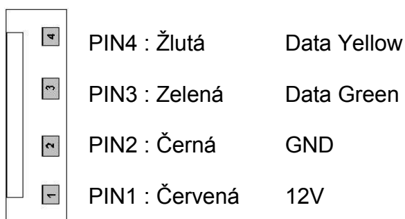
Obrázek 4: Zapojení konektoru PROGRAM
